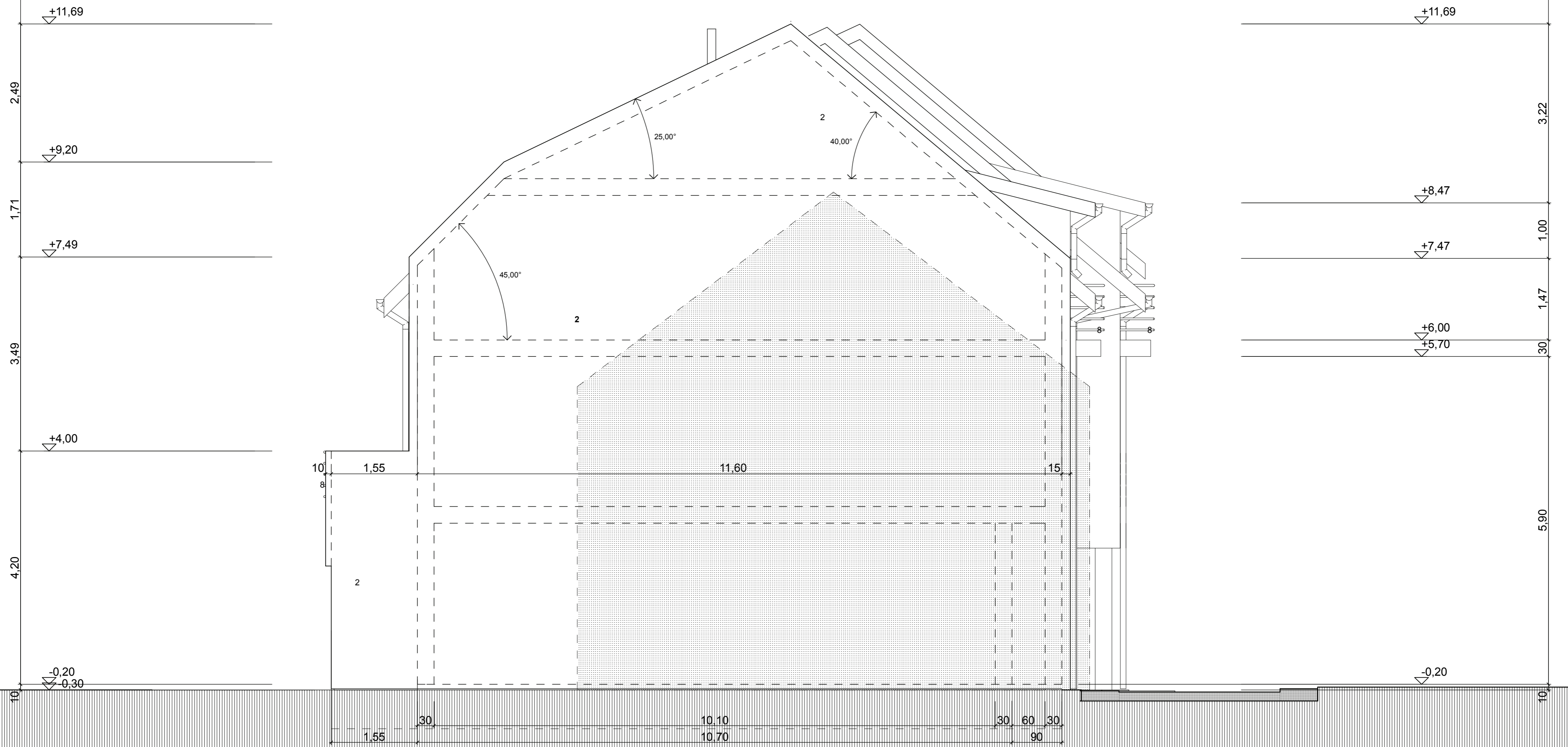
déli homlokzat m= 1: 100
