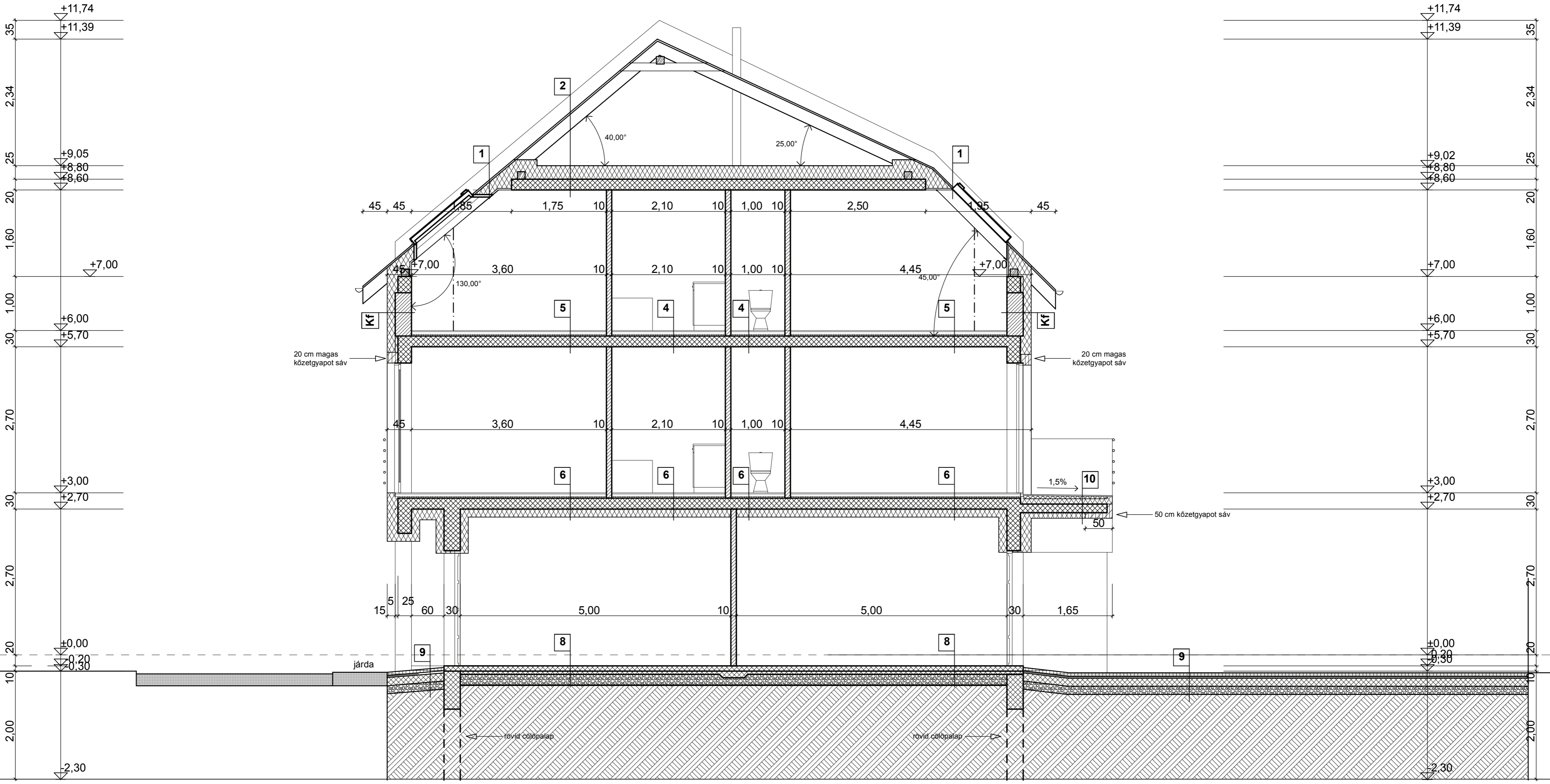
A-A metszet m= 1: 100
