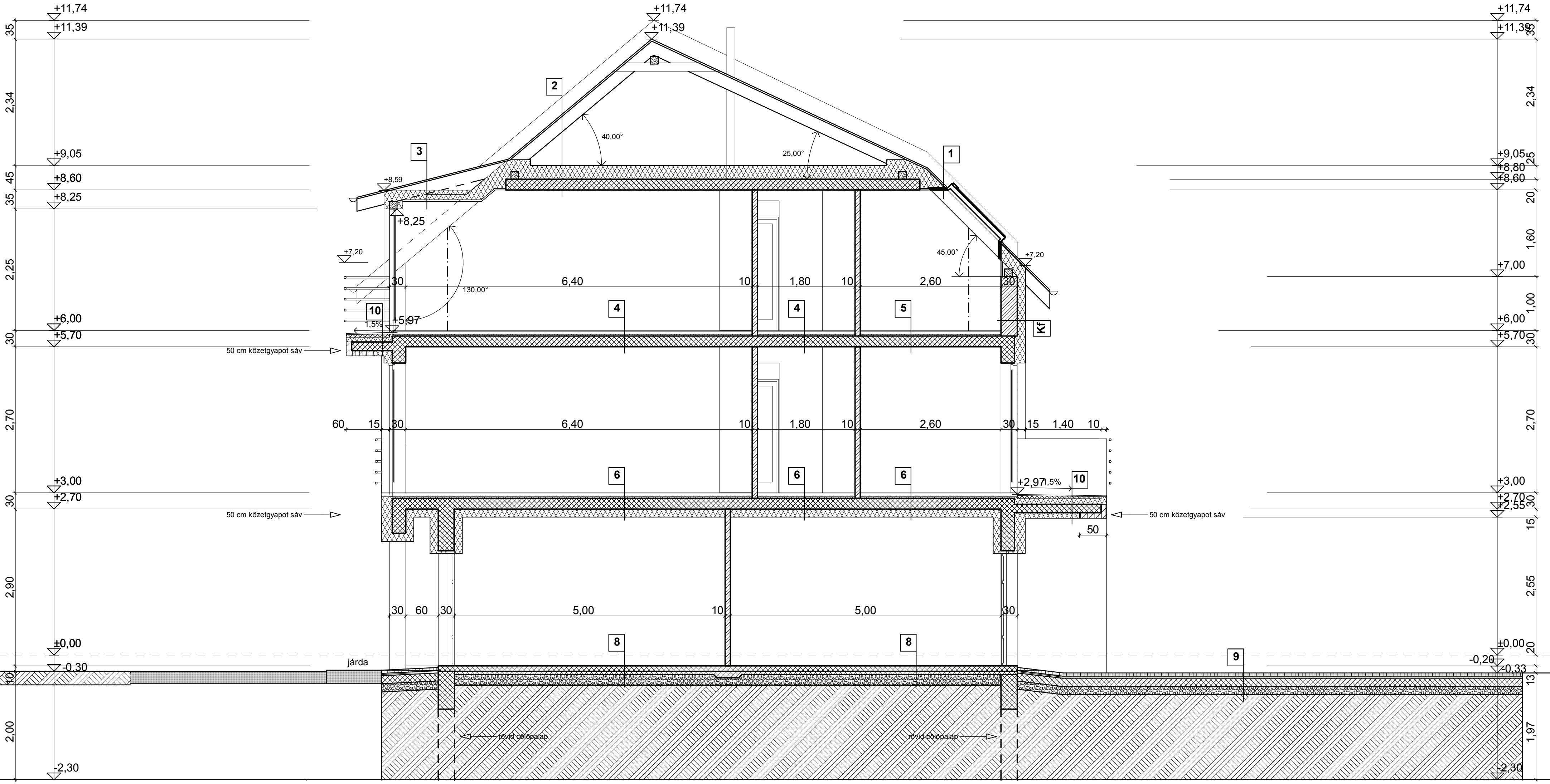
B-B metszet m= 1: 100
