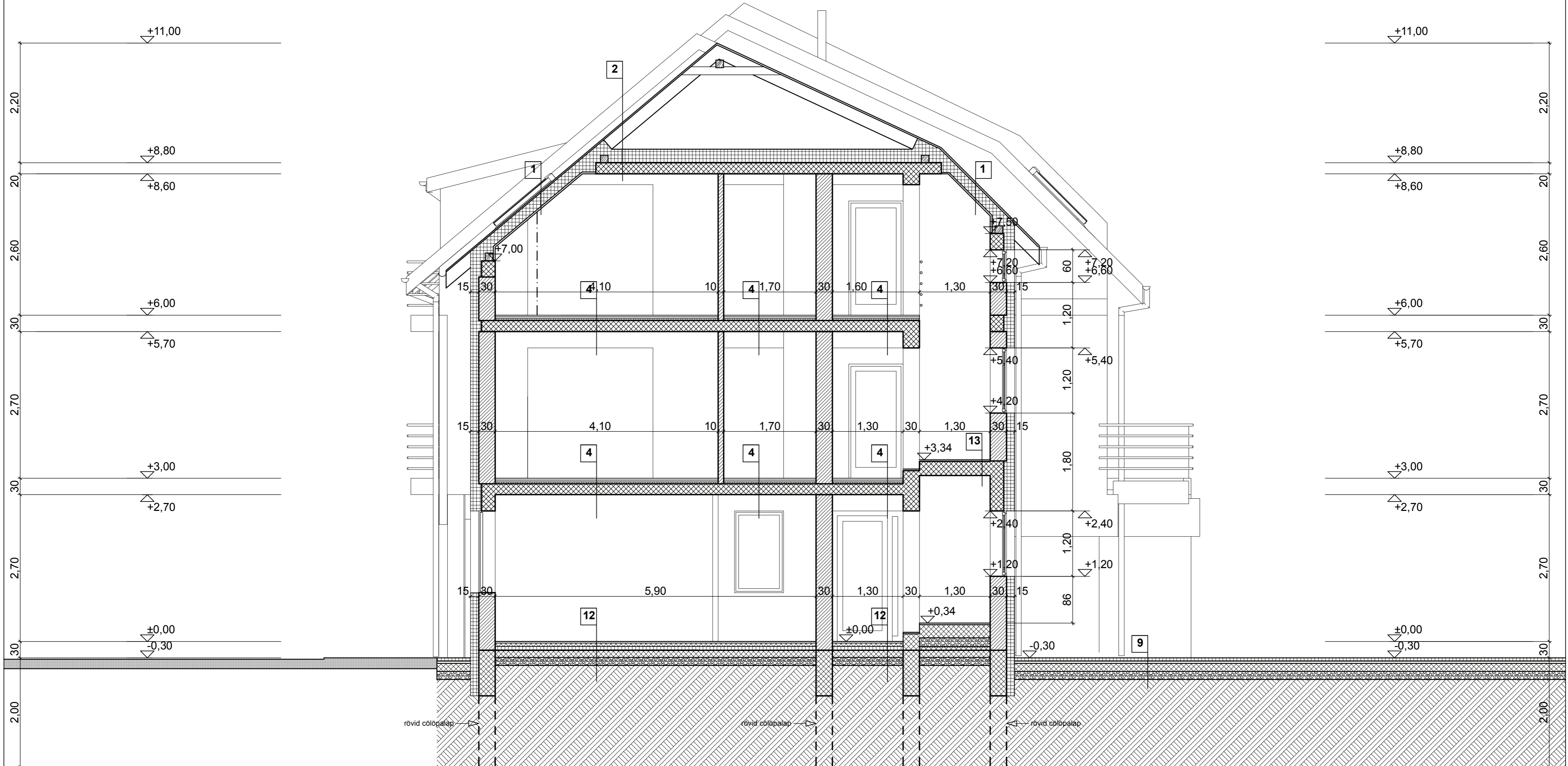
C-C metszet m= 1: 100
