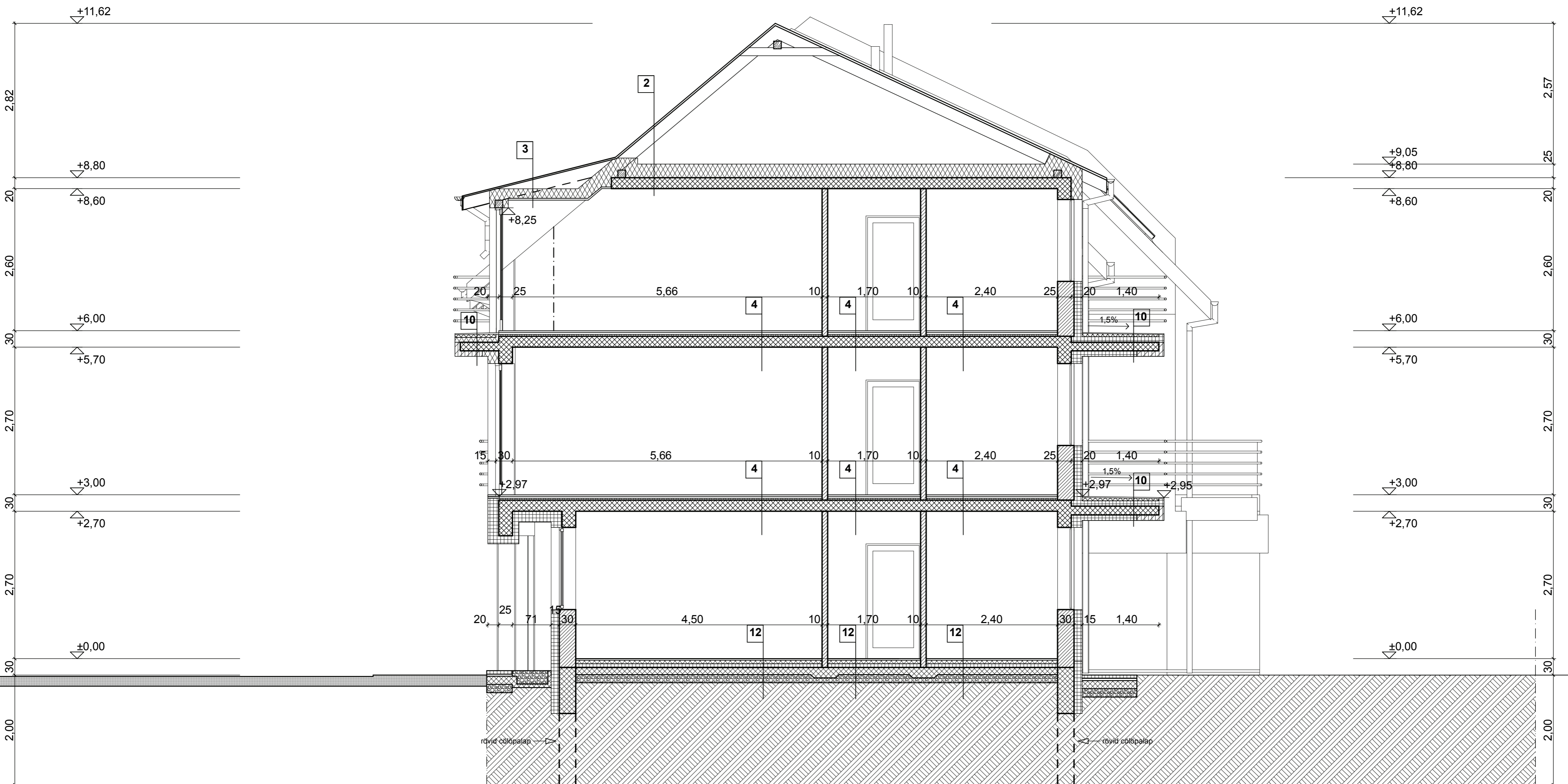
D-D metszet m= 1: 100
