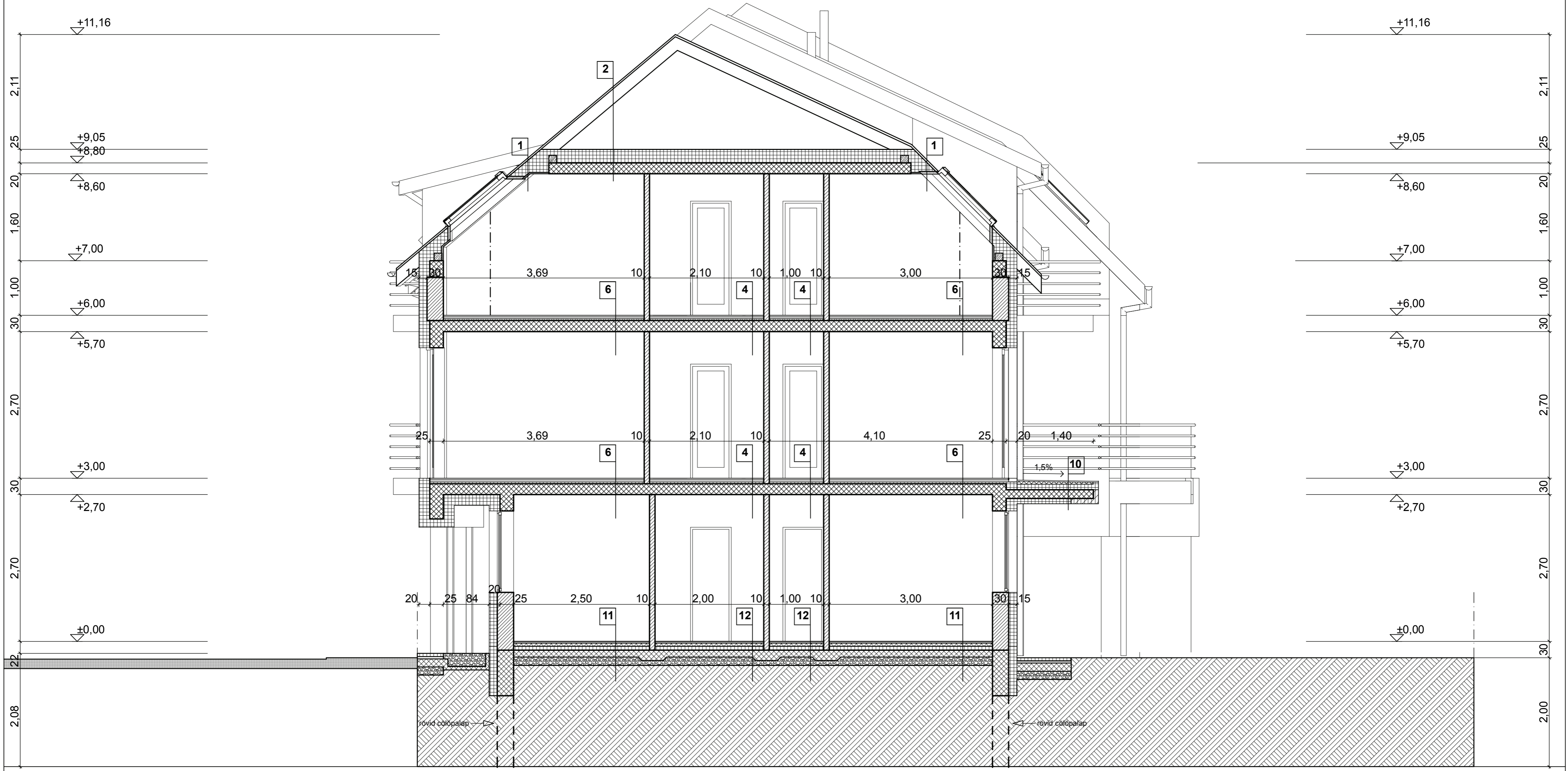
E-E metszet m= 1: 100
